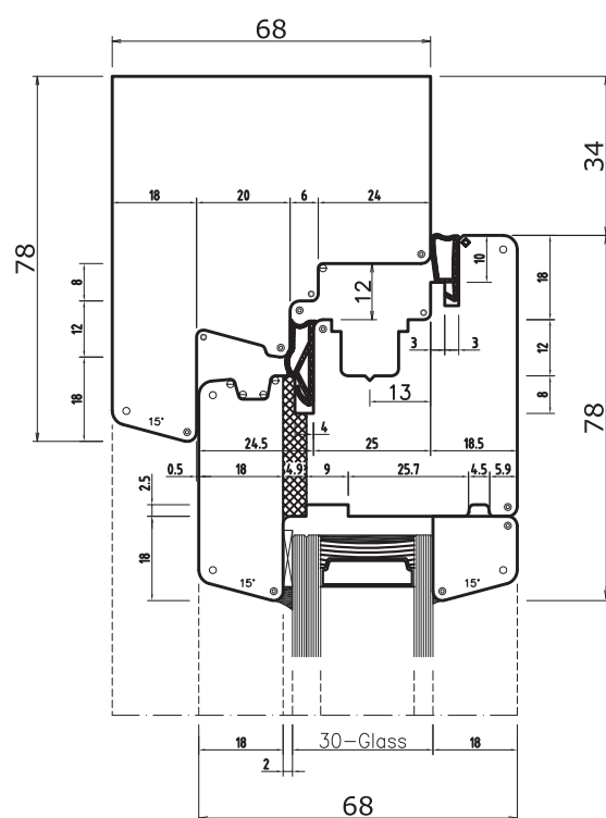
Secţiune verticală
