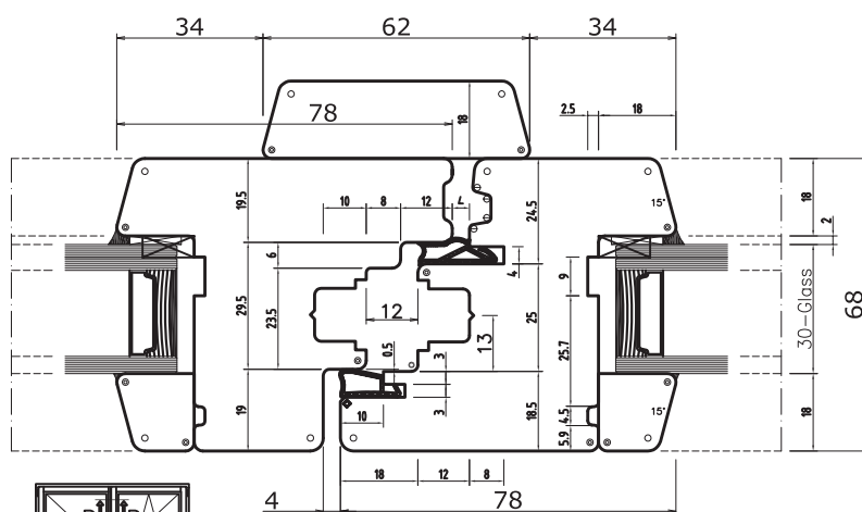
Secţiune verticală
