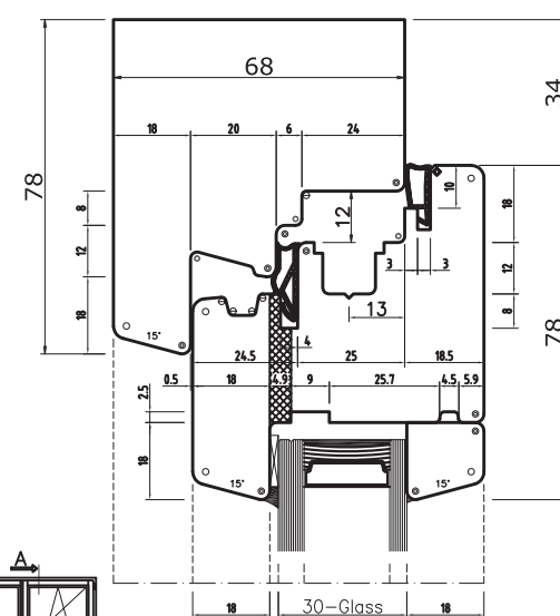
Secţiune verticală
